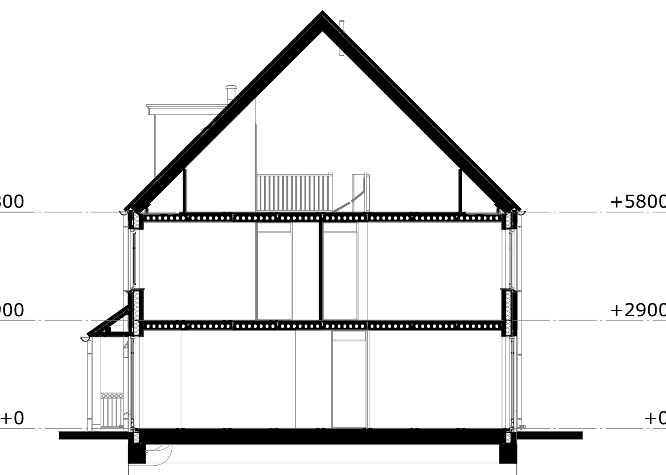
doorsnede B
