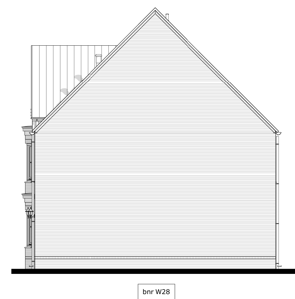
rechter zijgevel
