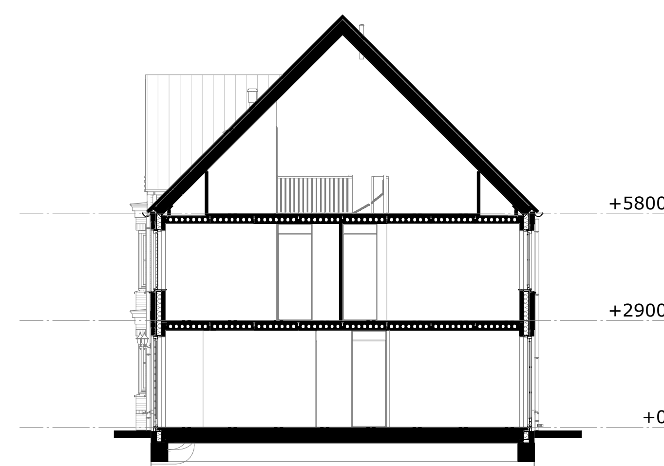
doorsnede B
