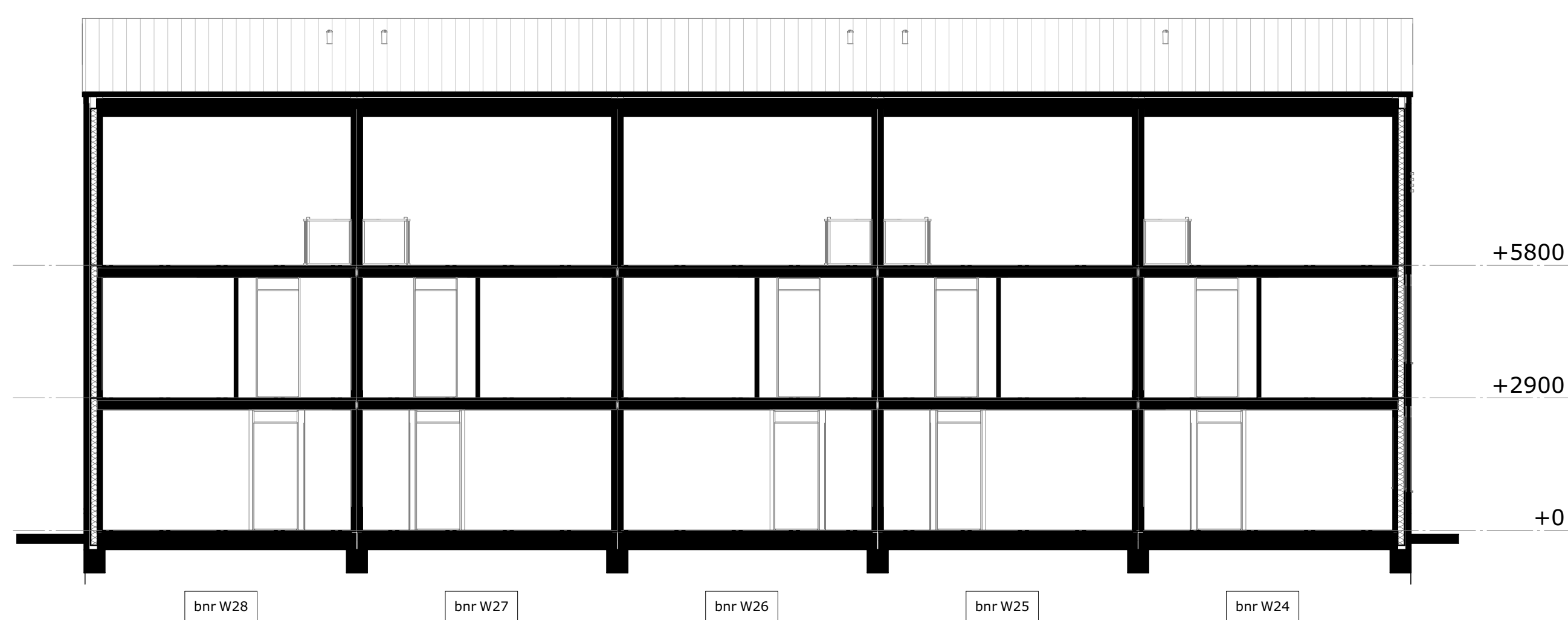
doorsnede A
