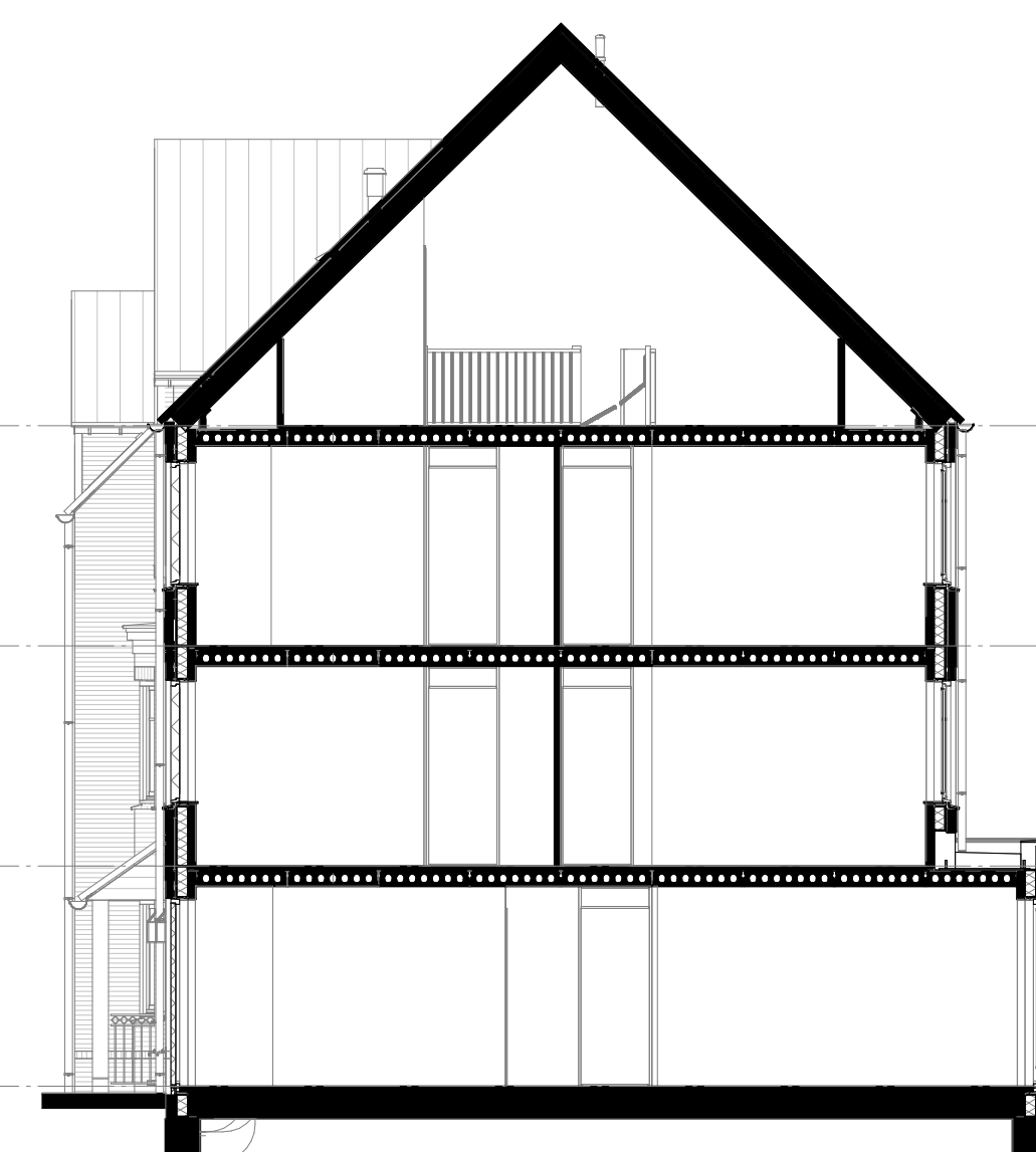
doorsnede B
