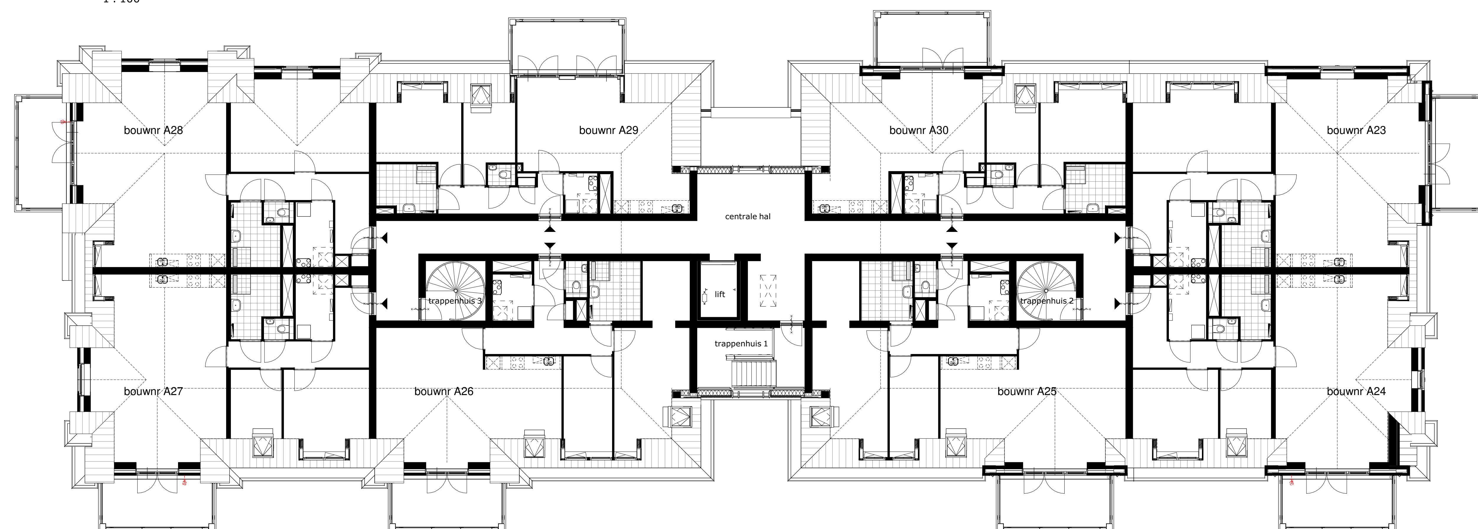
derde verdieping 1 : 100
