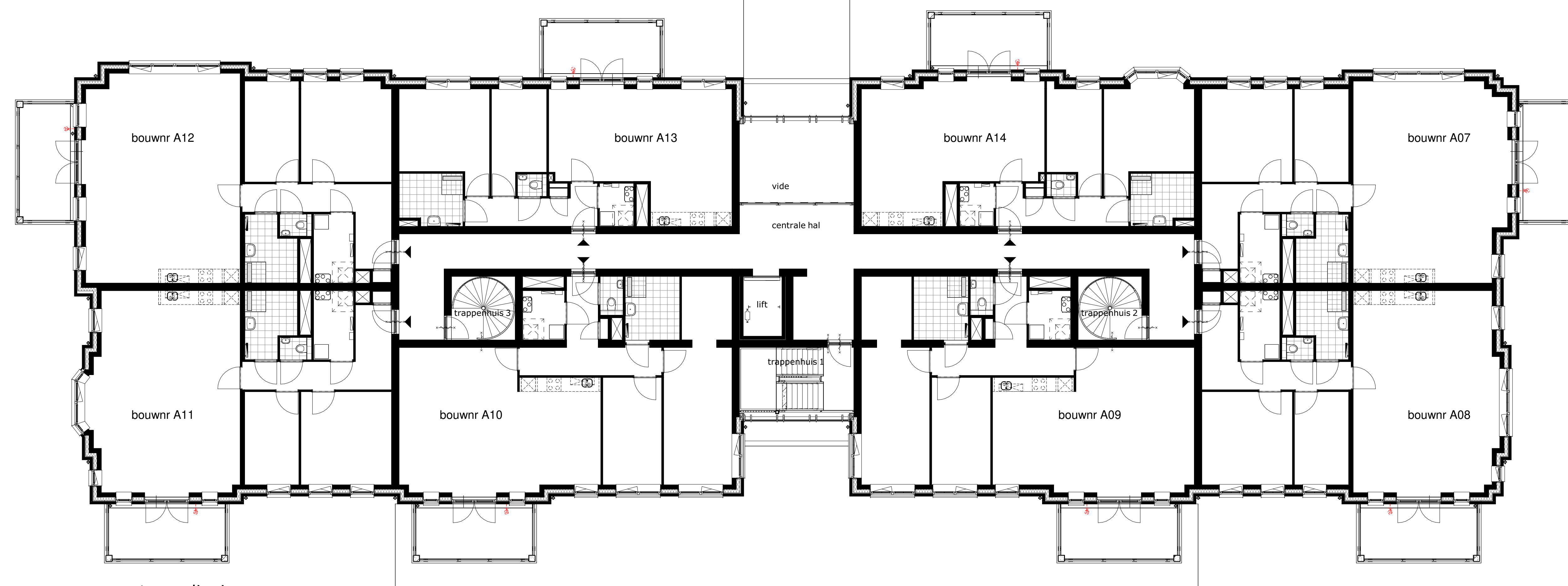
eerste verdieping 1 : 100
